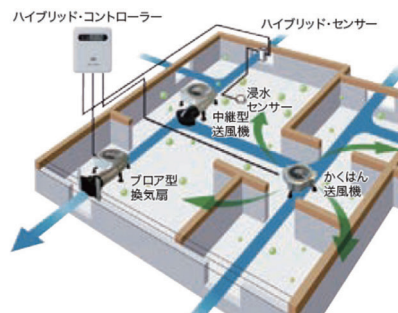
床下換気イメージ
